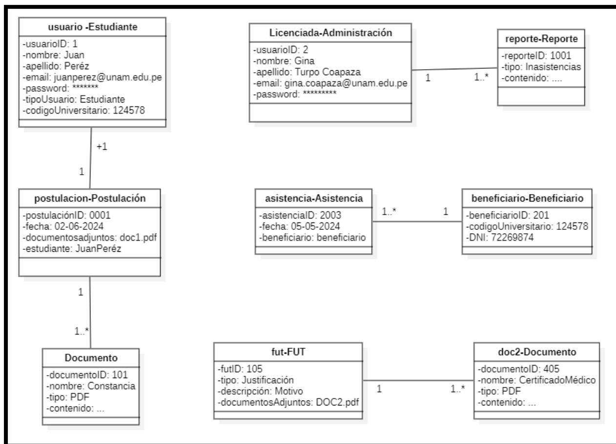
Diagrama 22: Objeto
