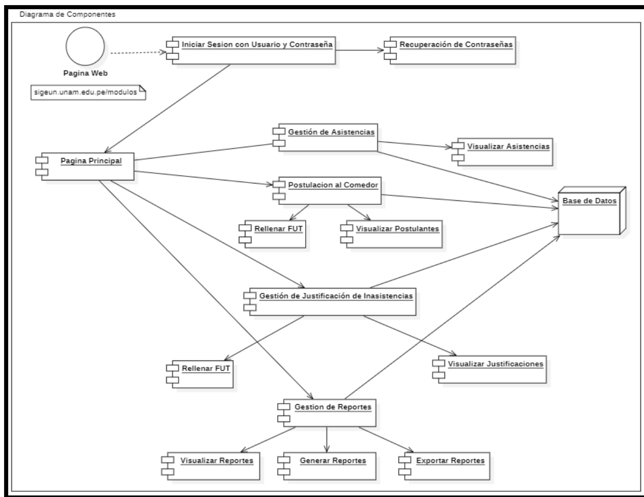
Diagrama 23: Componentes
