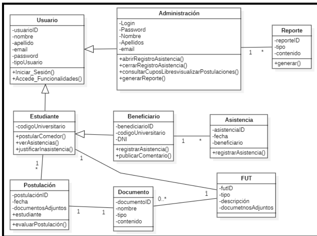
Diagrama 20: Clases
