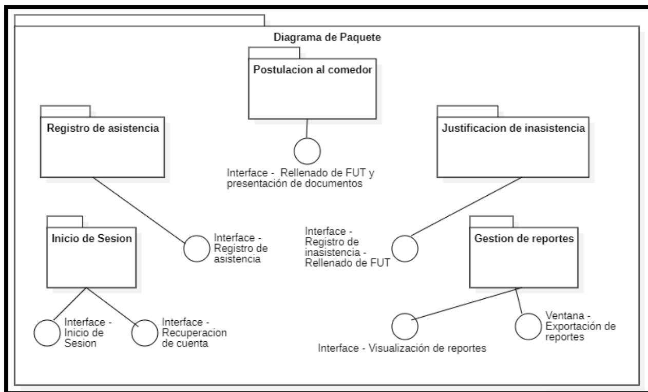
Diagrama 21: Paquete
